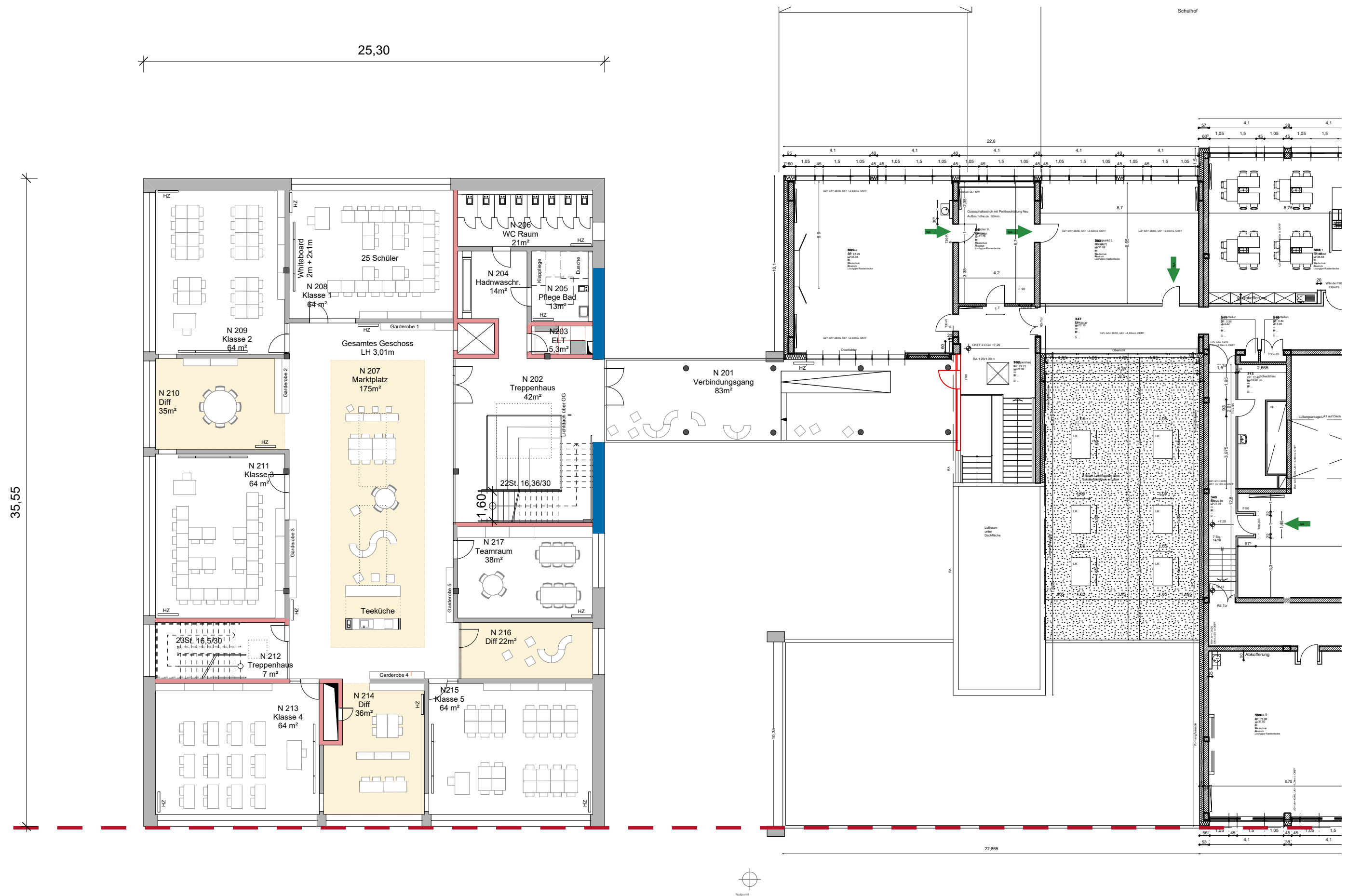
Neubau an der Oberschule Roter Sand Vorentwurf - 2. Obergeschoss
