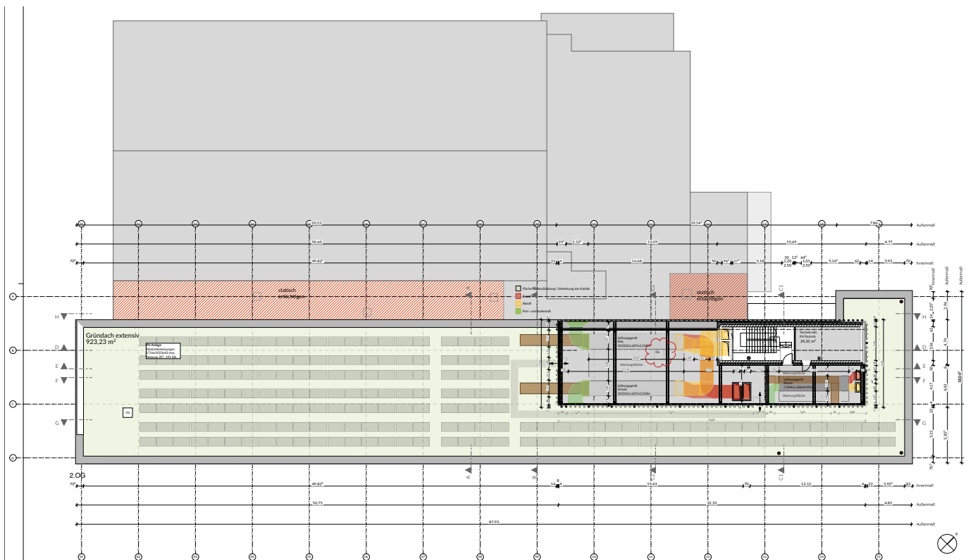
Grundriss 2.OG
