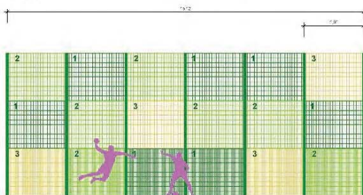
Ansicht Ballfangzaun Stirnseite Sportfeld 1 Richtung Schulstraße - H 6m M 1:50
