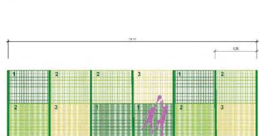
Ansicht Ballfangzaun Stirnseite Sportfeld 1 Richtung Friedrich-Ebert-Straße - H 4m M 1:50
