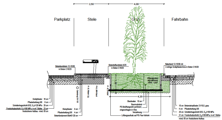
Querschnitt 3-3
