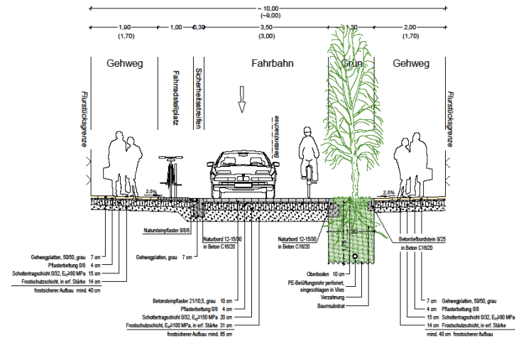
Querschnitt 1 Georg-Droste-Straße (Nollendorfer Straße)
